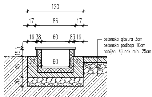
uzdužni presjek
