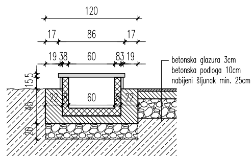
uzdužni presjek
