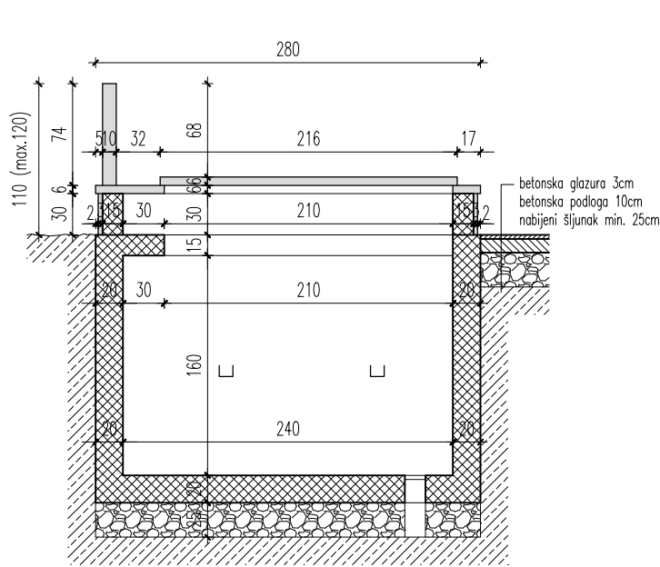
uzdužni presjek
