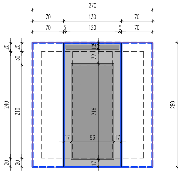
tlocrt
