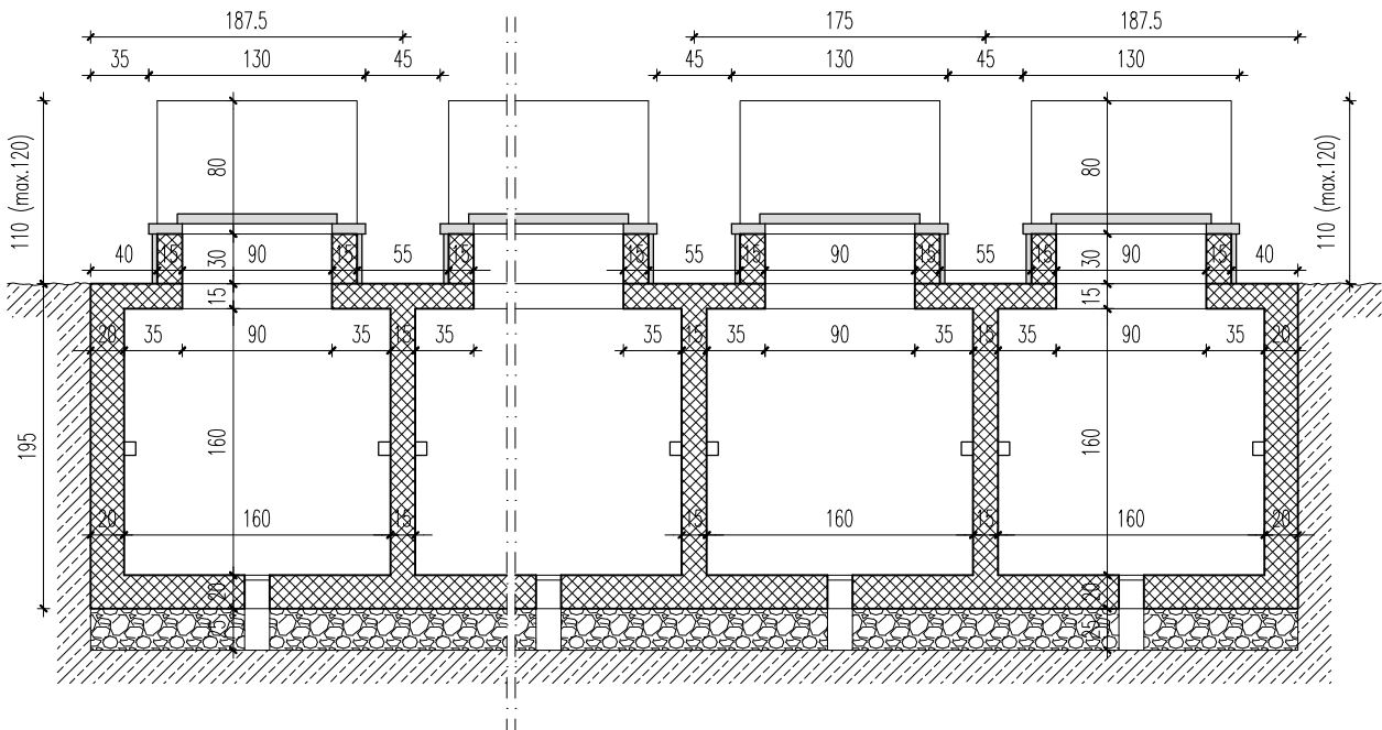
poprečni presjek
