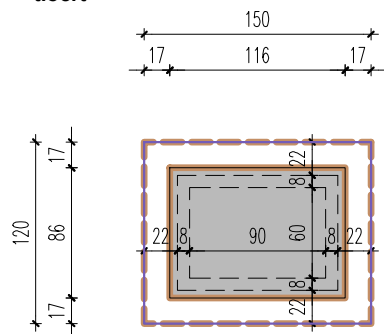
tlocrt
