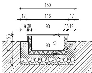
poprečni presjek
