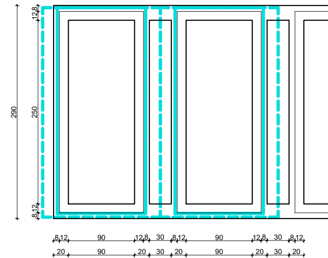
tlocrt
