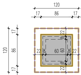
tlocrt
