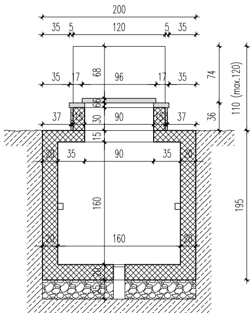
poprečni presjek
