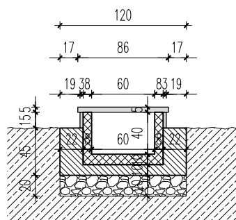
poprečni presjek
