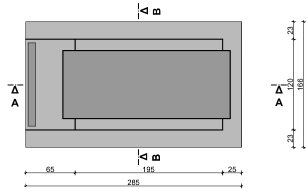
tlocrt
